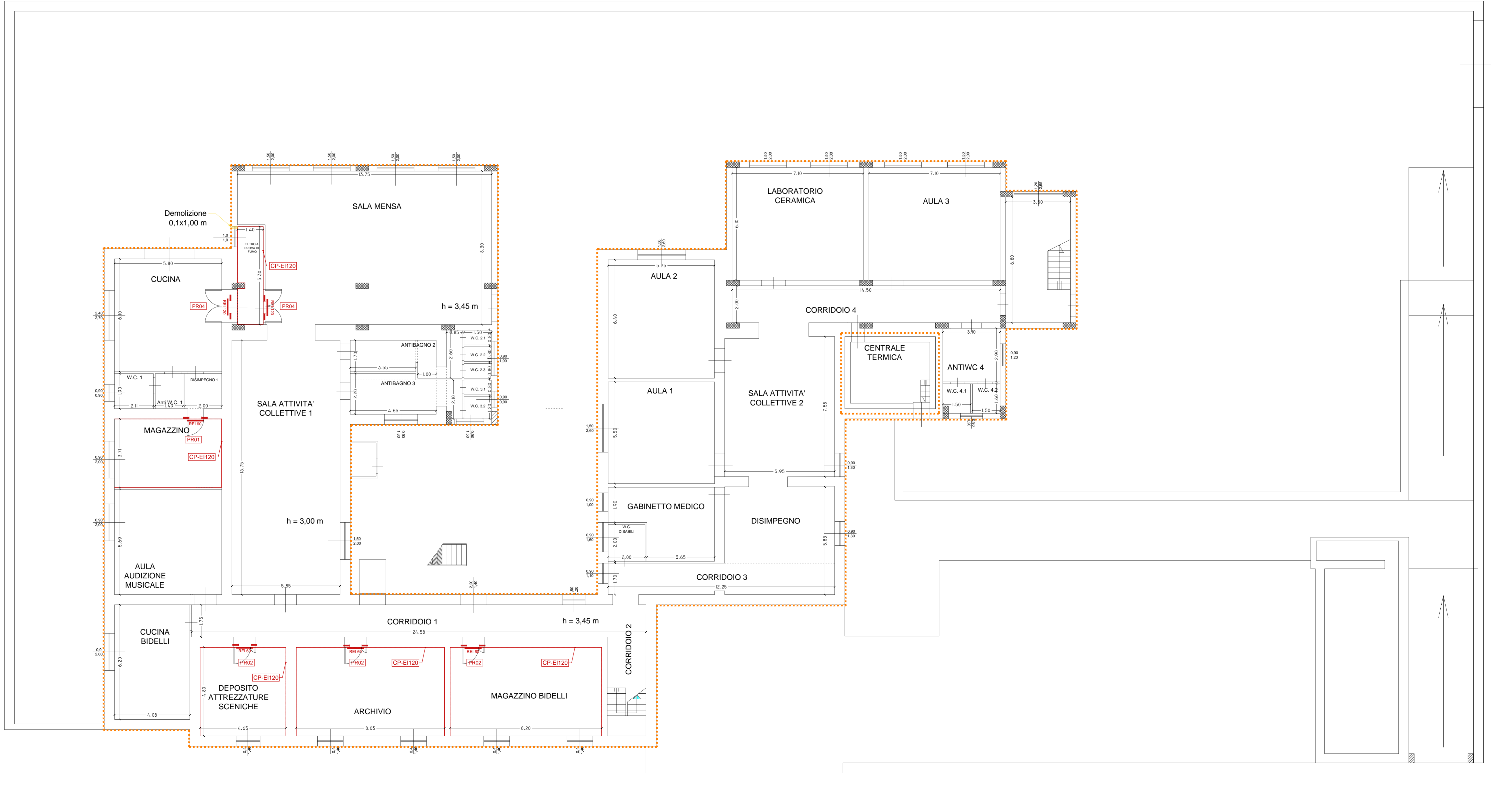
PIANTA PIANO SEMINTERRATO_SCALE 1:100
